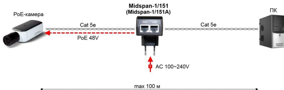
Рис. 3. Схема подключения инжекторов Midspan-1/151, Midspan-1/151A
